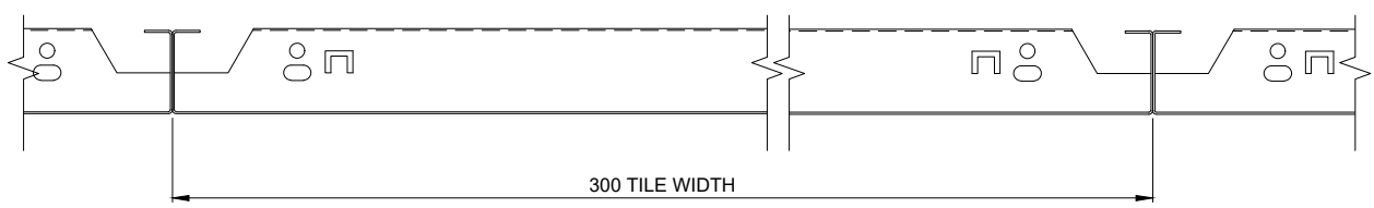
SECTION 'B'
