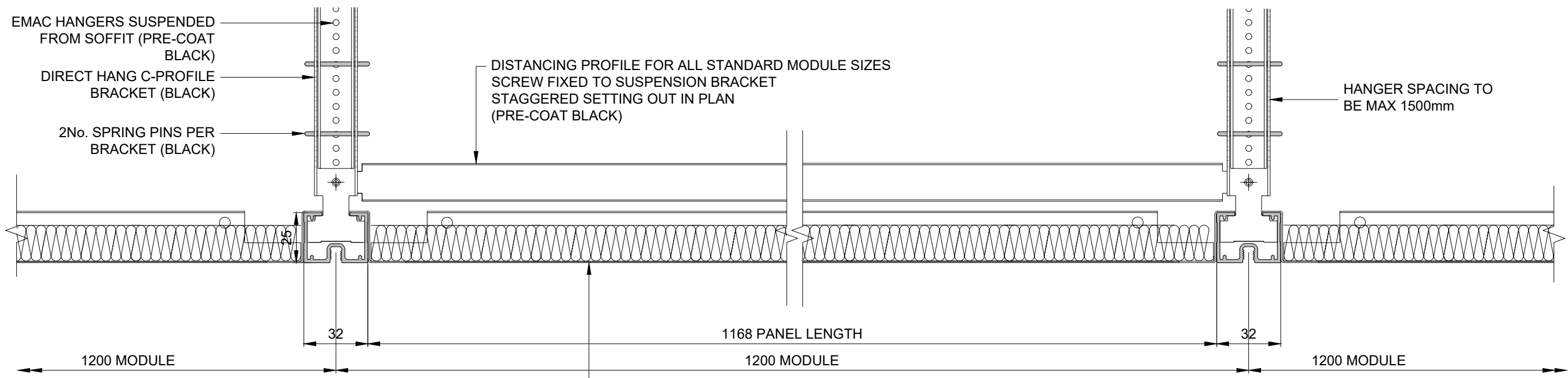
SECTION 'A'
