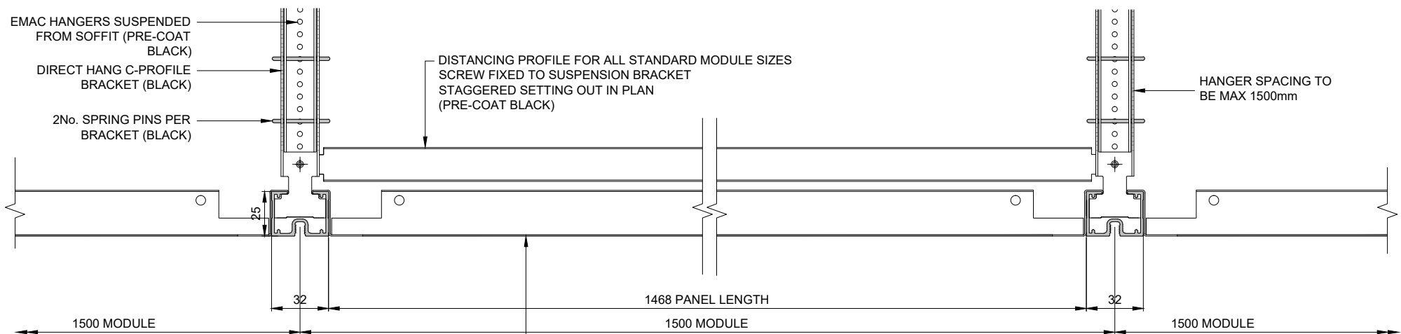
SECTION 'A'
